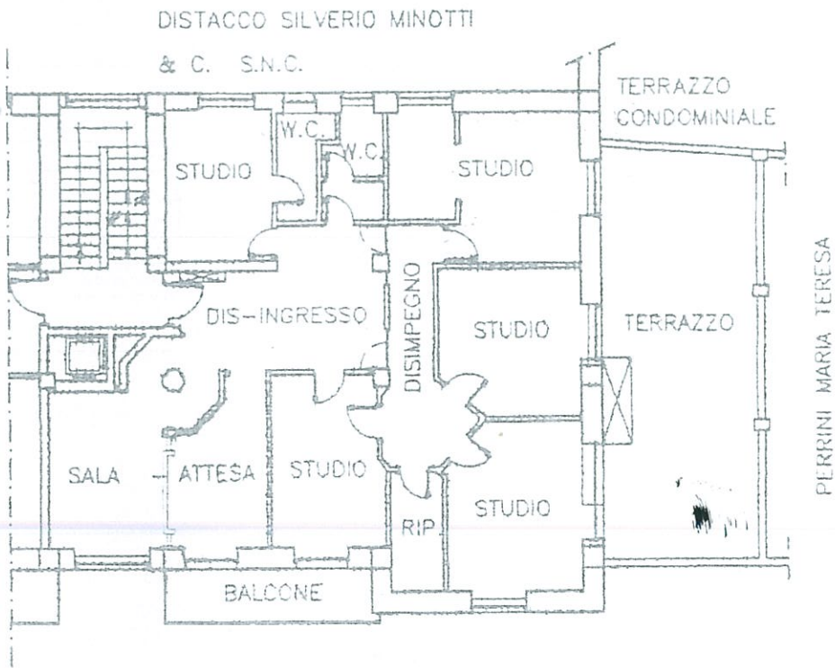
PIANO PRIMO H=3,10 ml.
